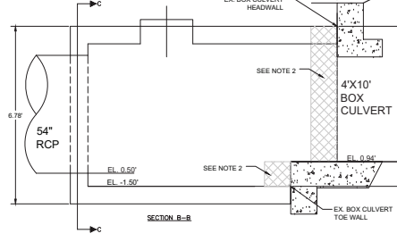
Manhole MH-6 - Sta. 66+61.45
